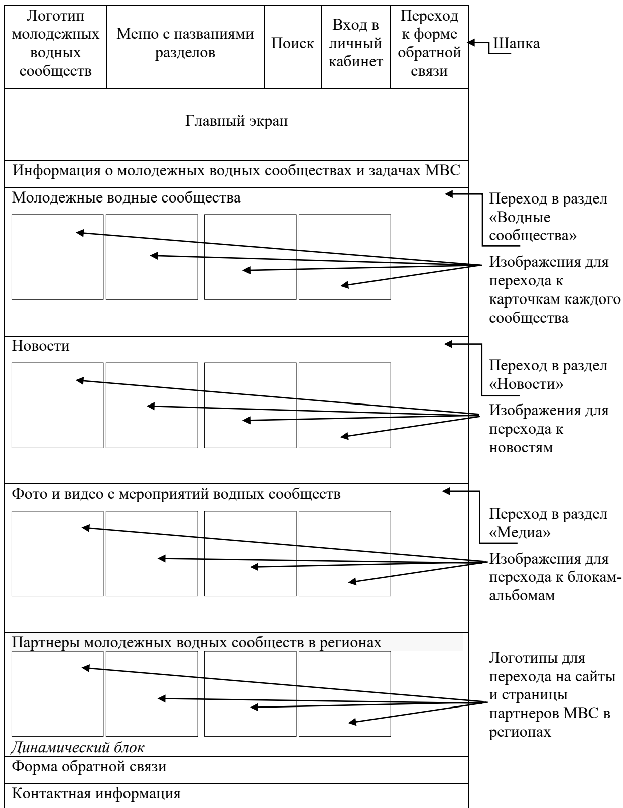
Рисунок 1. Схема главной страницы-лендинга сайта водные сообщества.рф
